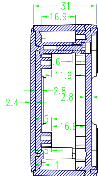
SEC D-D
