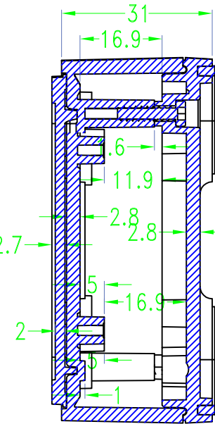
SEC D-D
