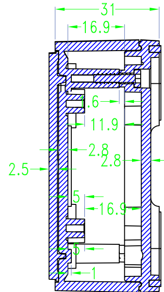
SEC D-D
