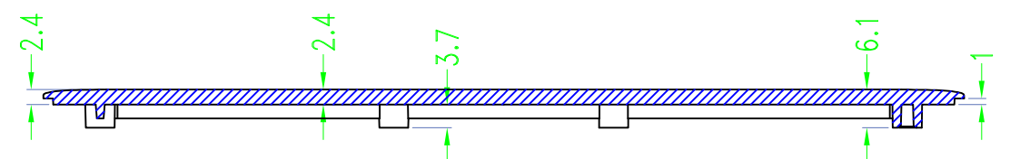
SEC A-A
