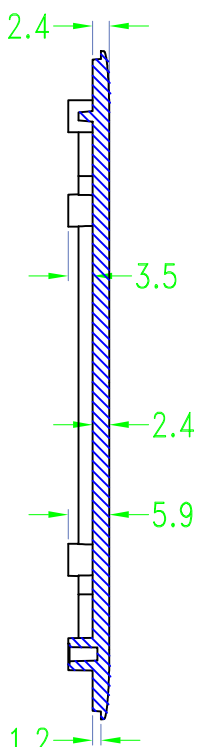
SEC A-A
