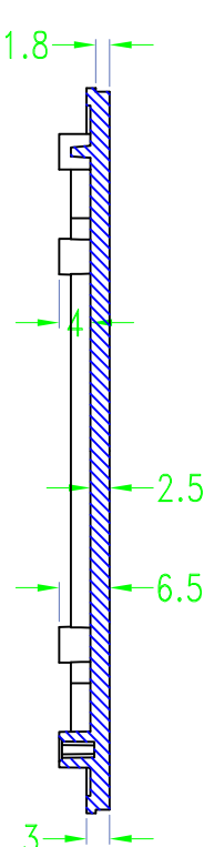
SEC A-A
