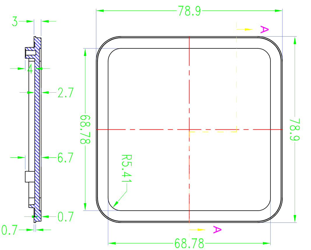
SEC A-A
