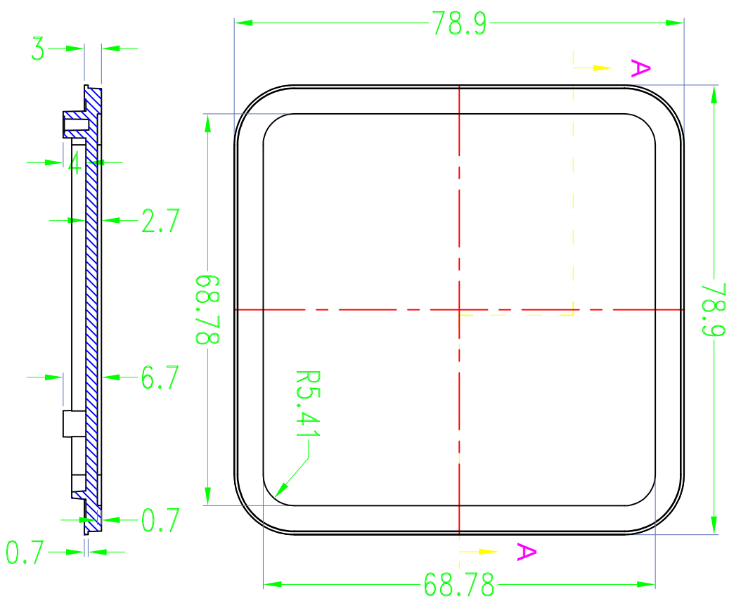
SEC A-A
