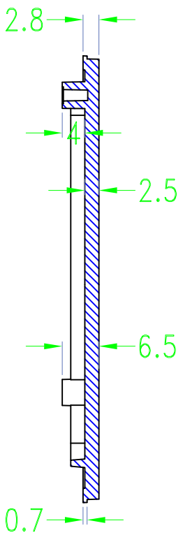
SEC A-A
