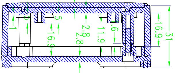
SEC D-D
