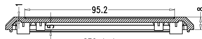
SEC A-A
