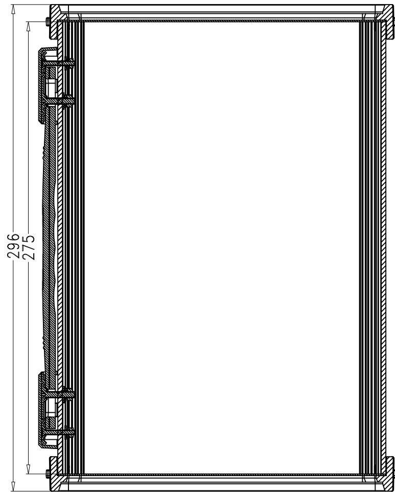
SEC A-A
