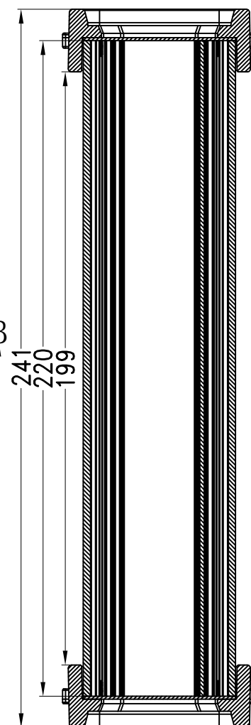
SEC A-A
