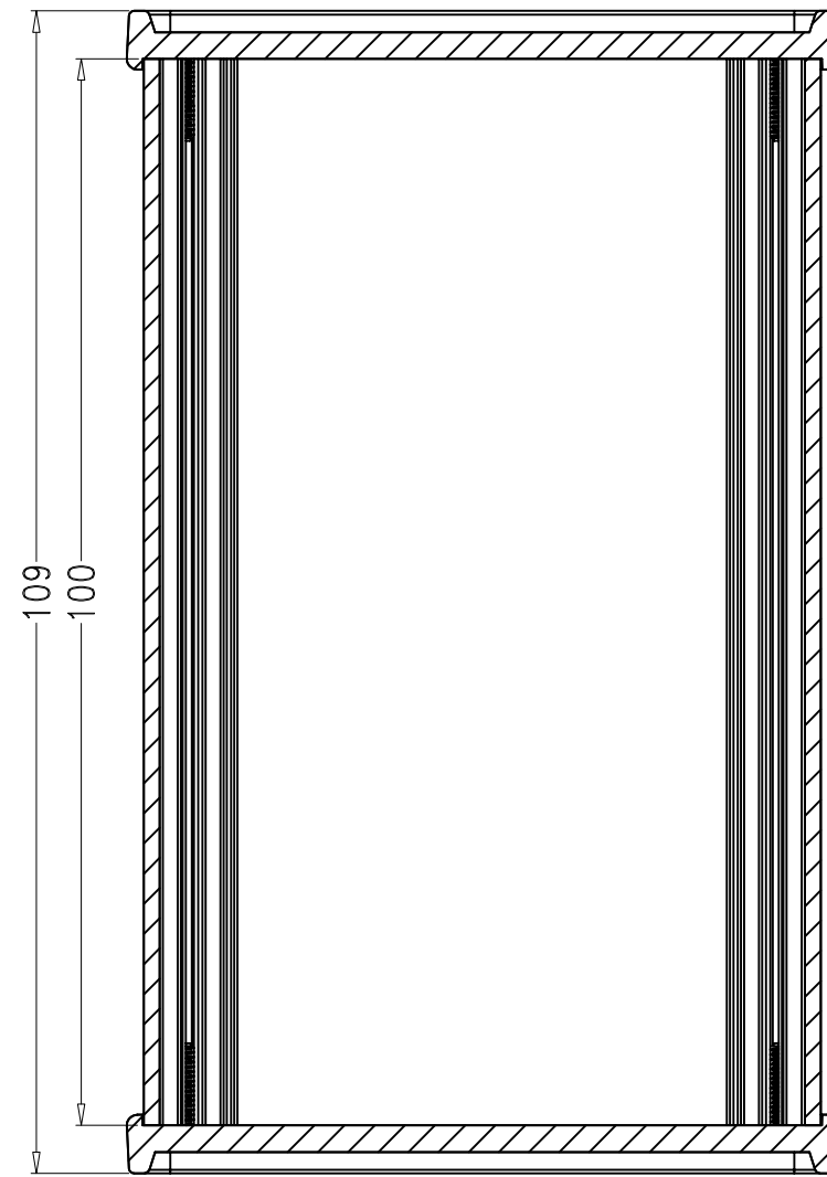
SEC A-A
