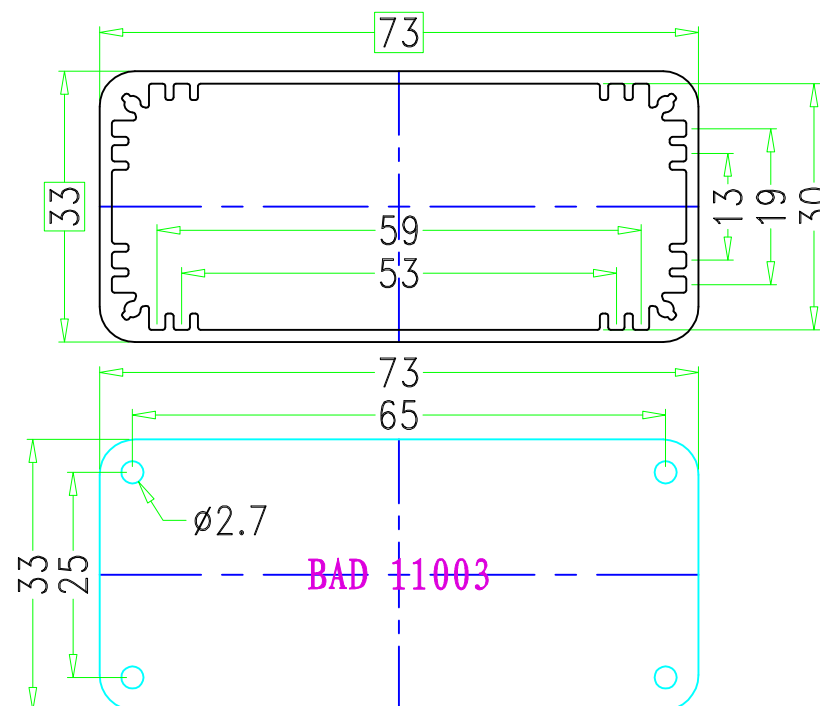
SEC A-A
