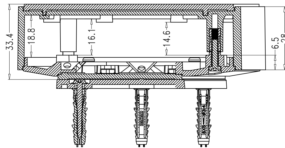
SEC A-A
