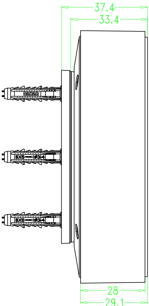
SEC A-A
