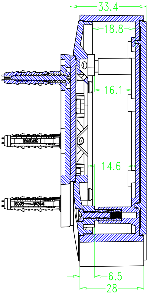
SEC A-A
