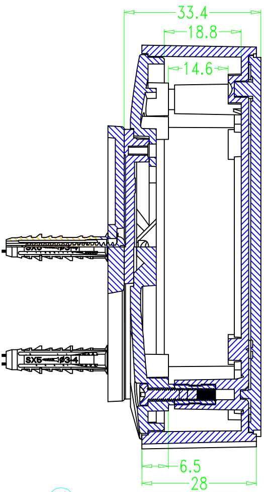
SEC A-A
