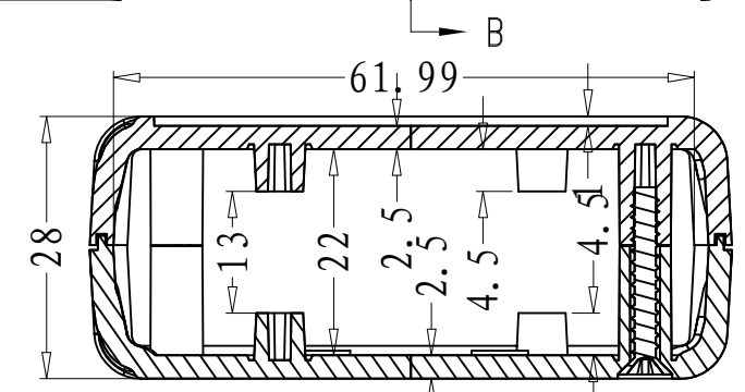
SEC A-A
