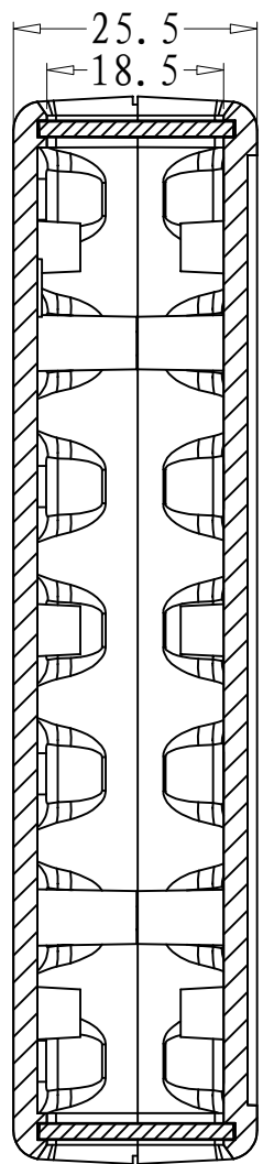
SEC A-A
