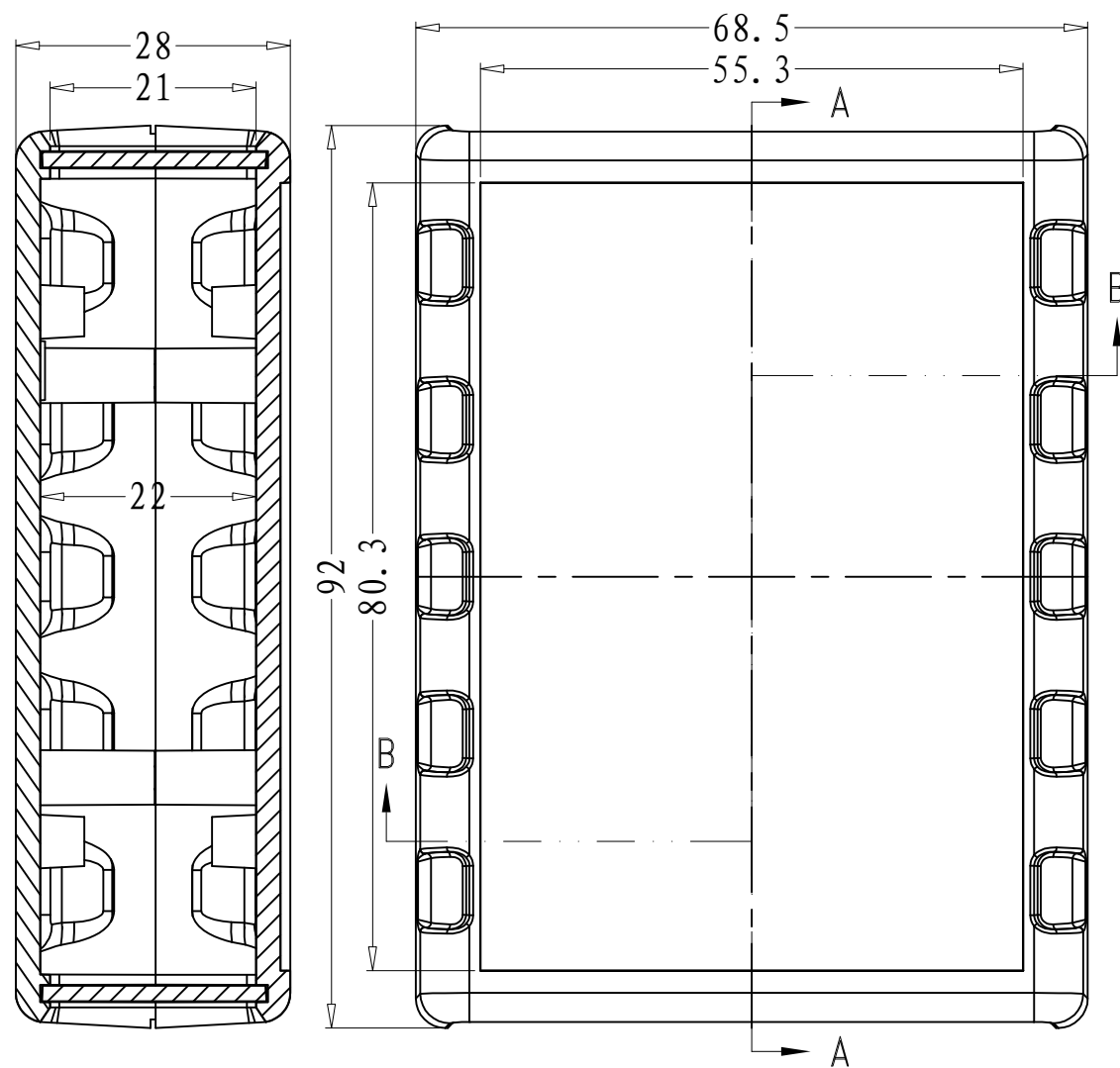
SEC A-A
